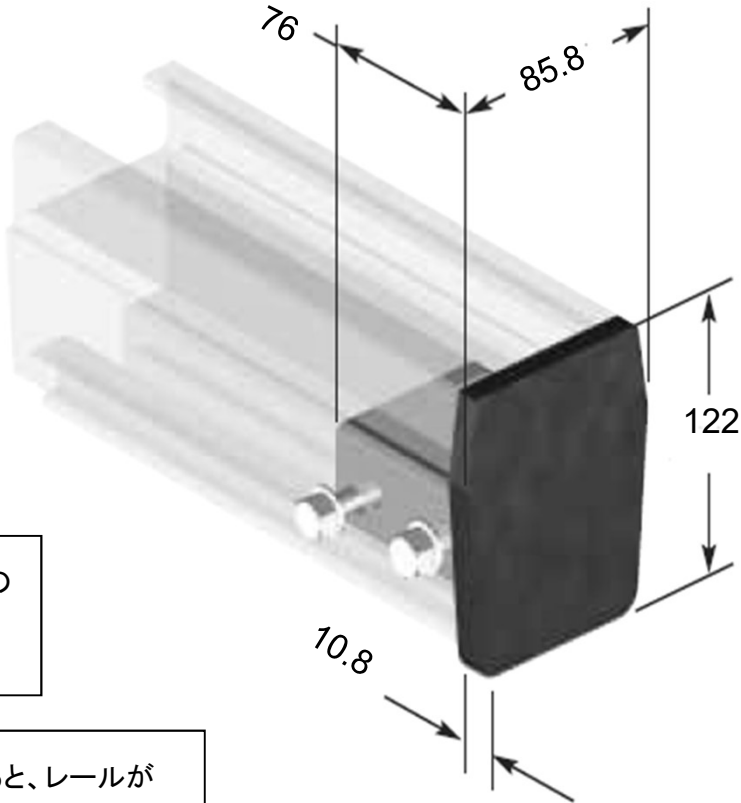
4インチレール寸法
